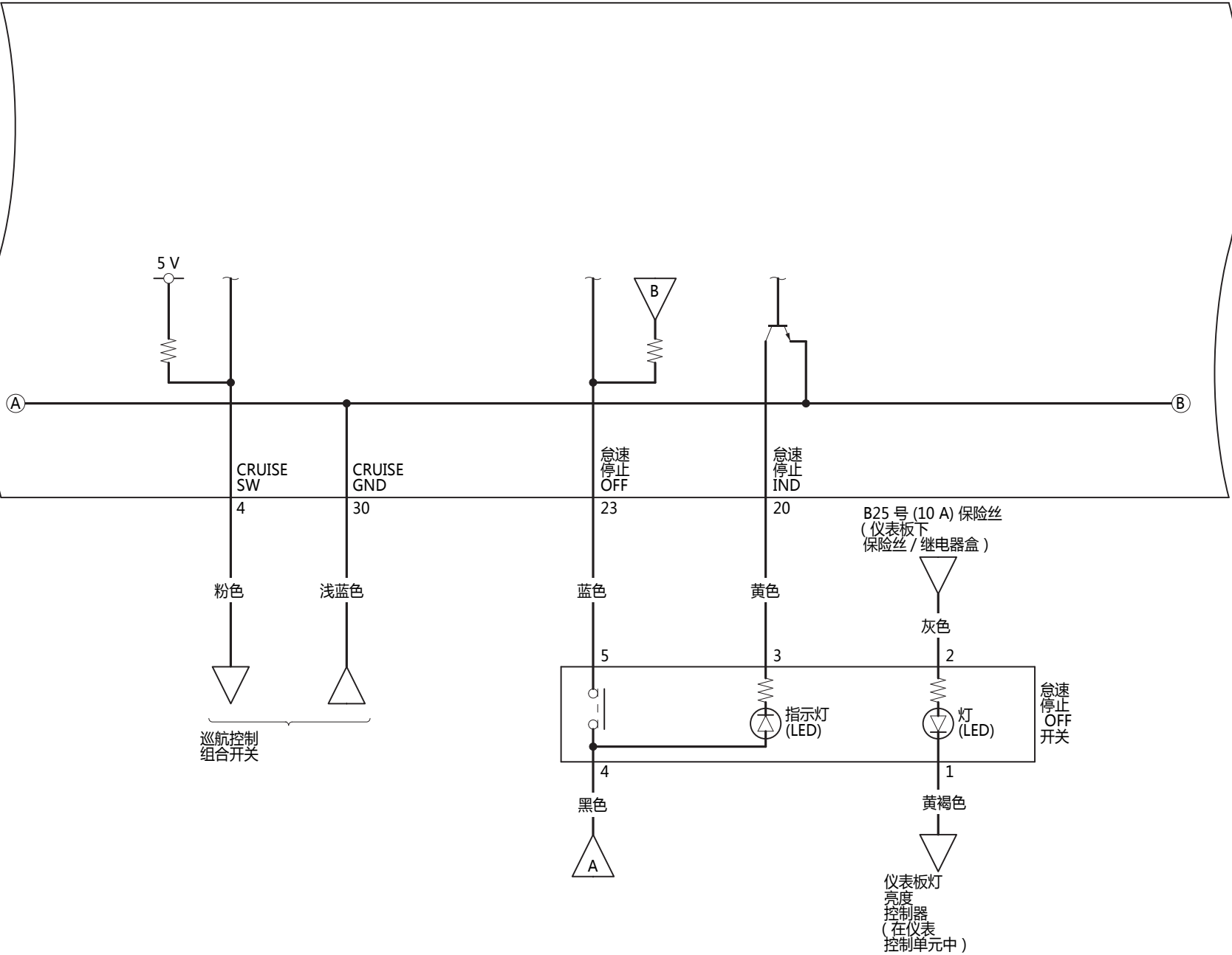
仪表控制单元
